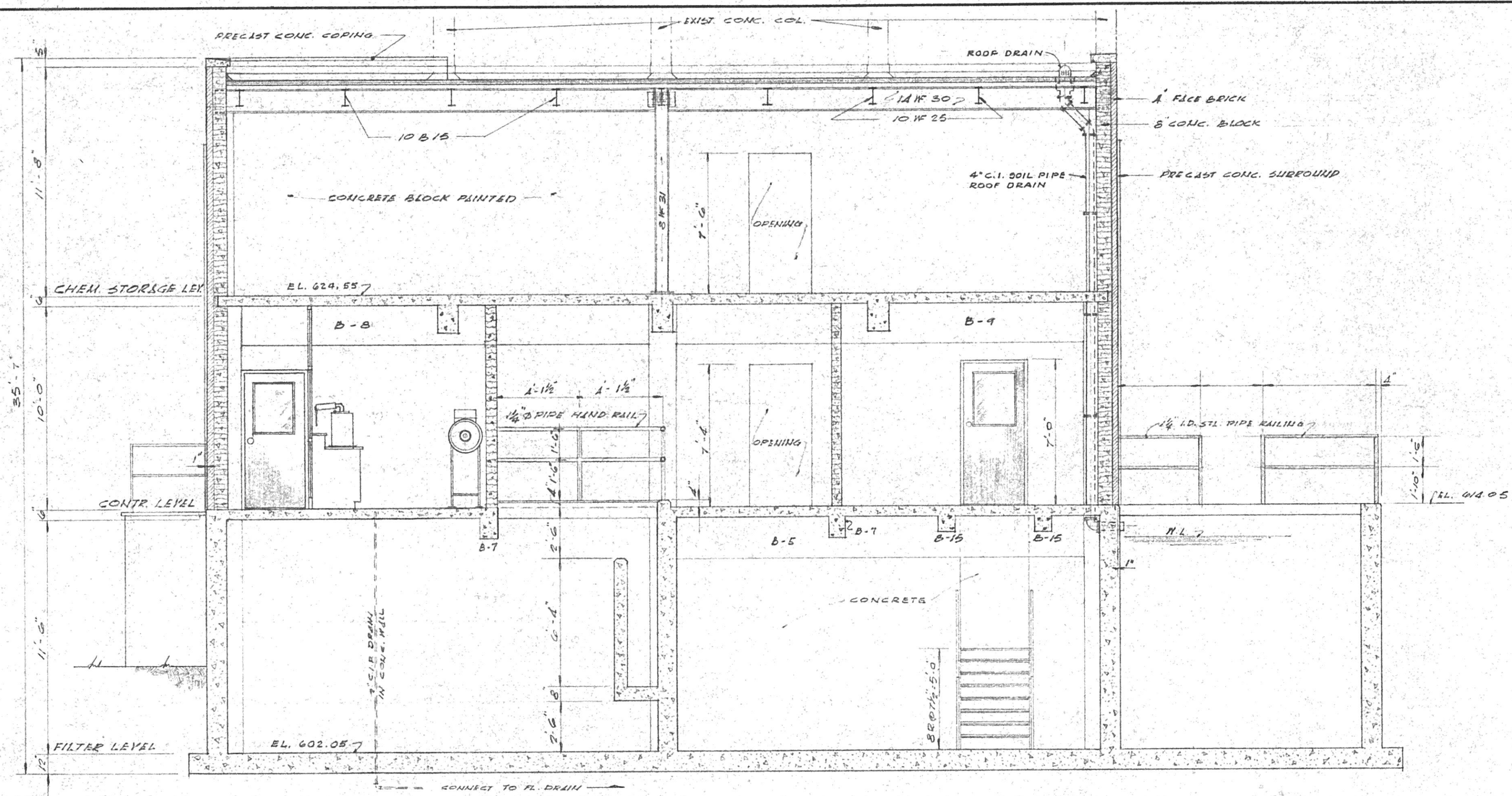
SECTION A-A SCALE: 1/4" = 1'-0"
